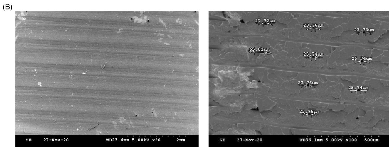
Raster angle 45°/- 45°, In-fill speed 35 mm/s
